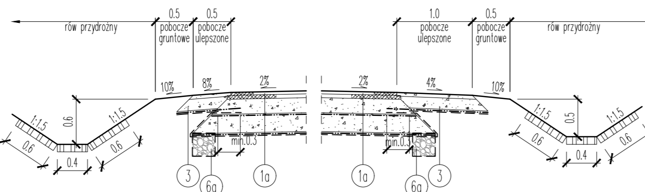
RÓW PRZYDROŻNY – UMCOENIE DŃA I SKARP
