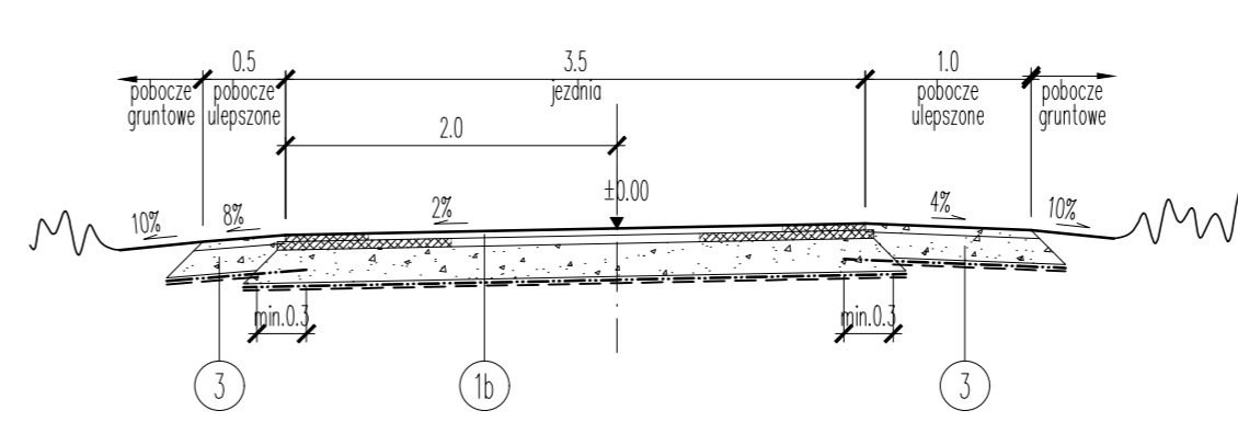
PRZEKROJE TYPOWE (km 0+351 ÷ ~0+740)
