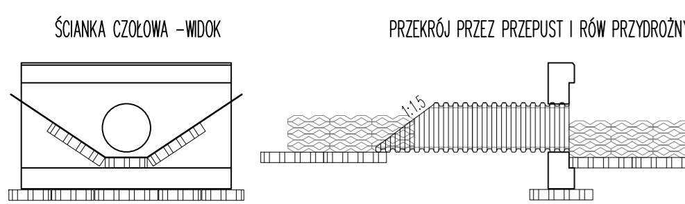
SCHEMAT ROZWIĄZAŃ PRZEPUSTÓW I UMCOENIĘ RÓWÓW PRZYDROŻNYCH
