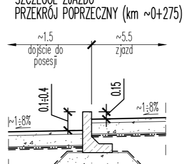
SZCZEGÓŁ ZJAZDU PRZEKÓJ POPRZECZNY (km ~0+275)
