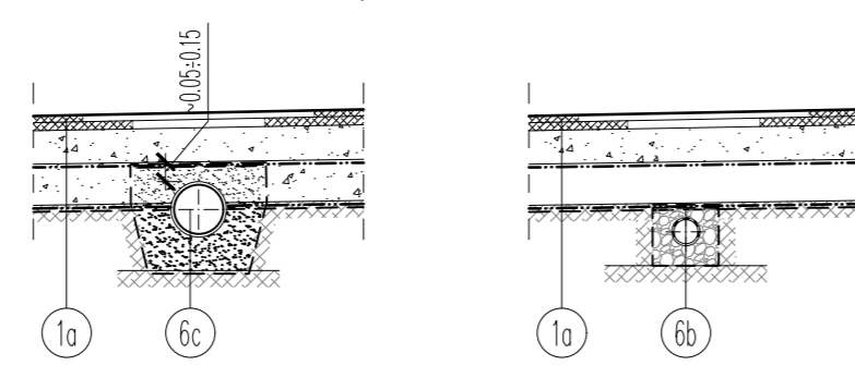
PRZEPUST I DRENAŻ POD KORONĄ DROGI
