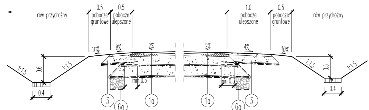
RÓW PRZYDROŻNY – UMCOENIE DŃA
