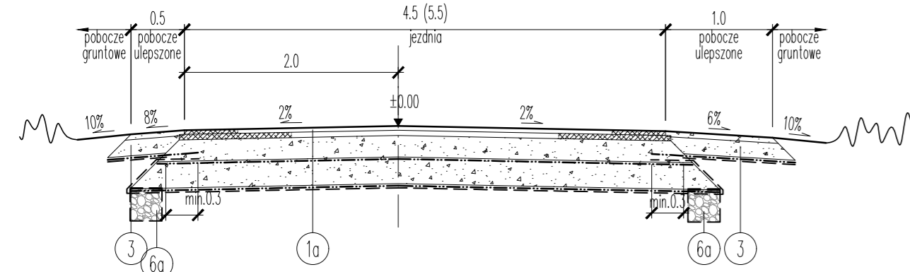
PRZEKROJE TYPOWE (km 0+007 ÷ 0+351)
