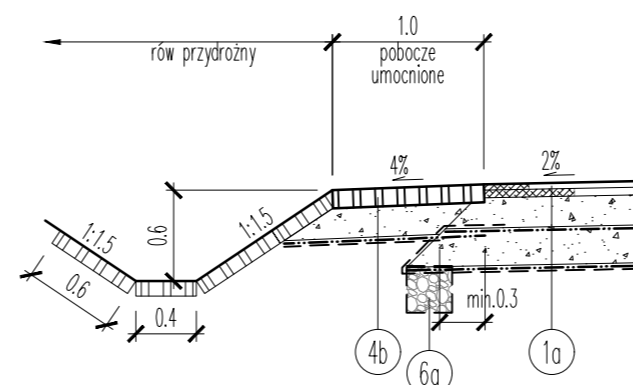
RÓW PRZYDROŻNY – UMCOENIE DŃA, SKARP I POCOBZA
